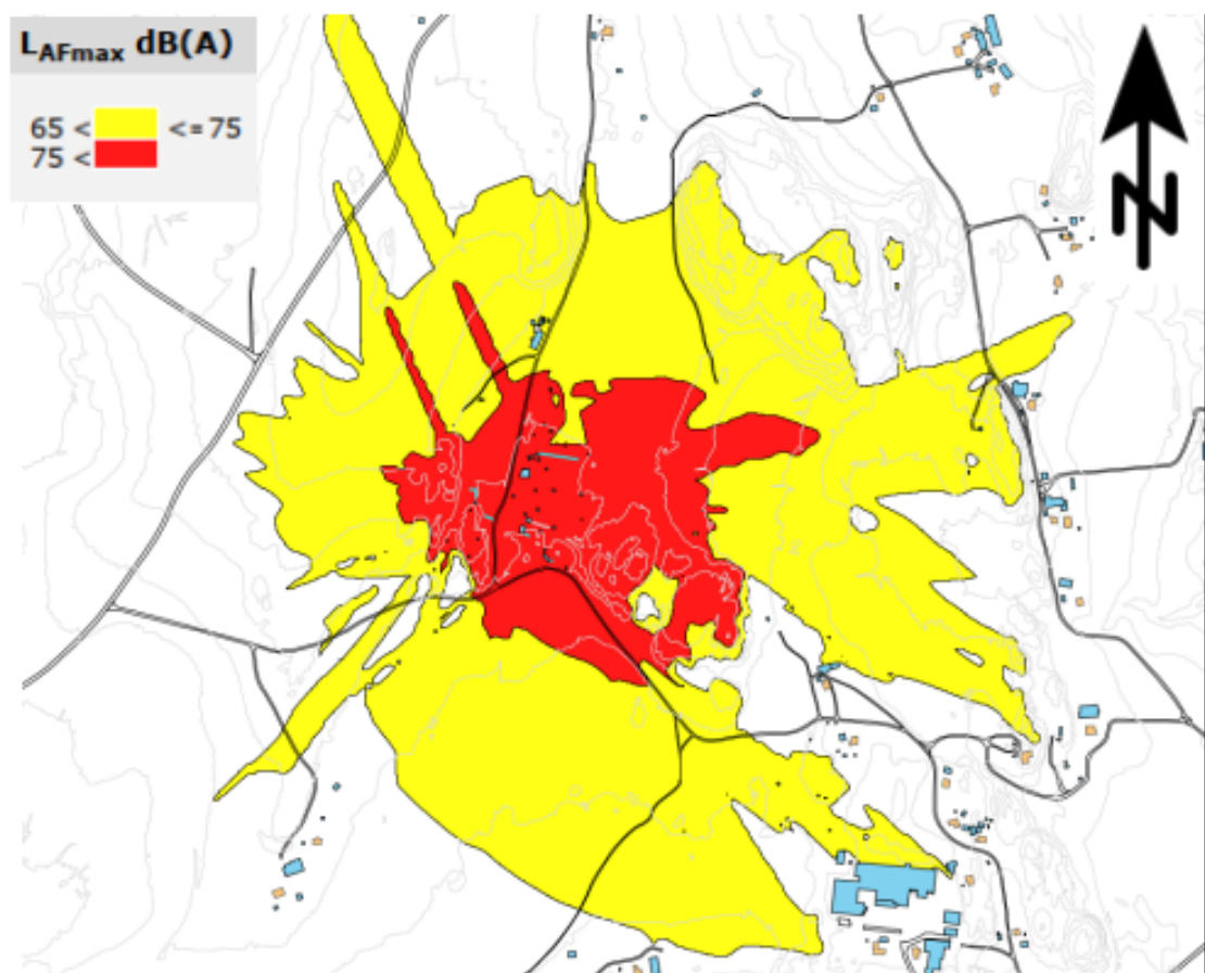
Figur 6 – Dolven skytebane. Støysoner basert på støygrenser for maksimalnivået.
