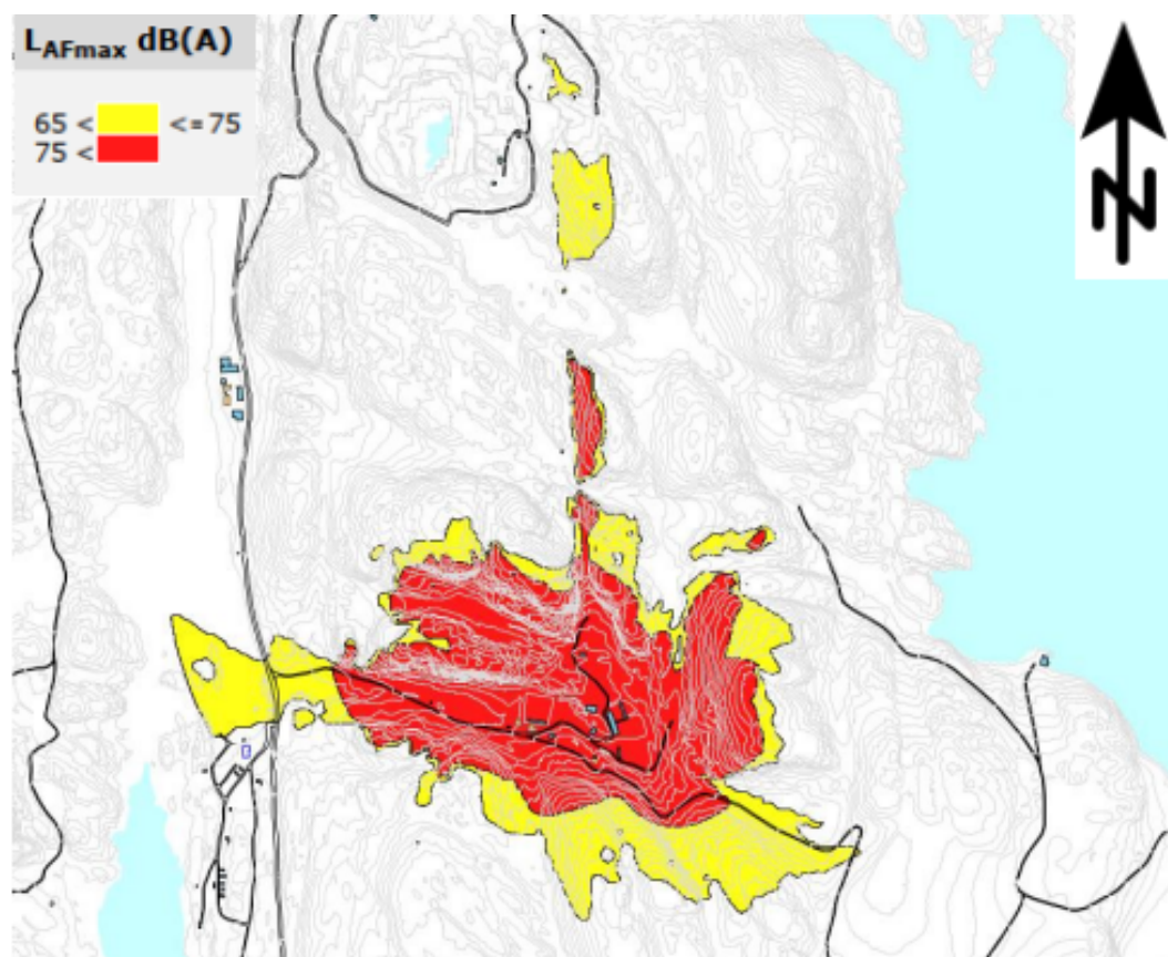
Figur 7 – Åres skytesenter. Støysoner basert på støygrenser for maksimalnivået.
